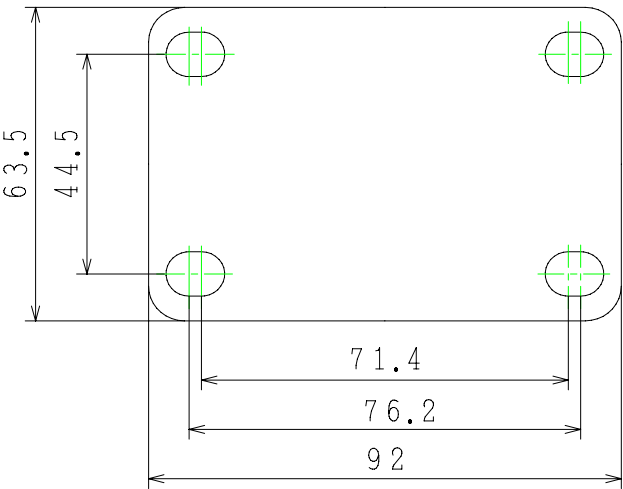
平板尺寸图：
