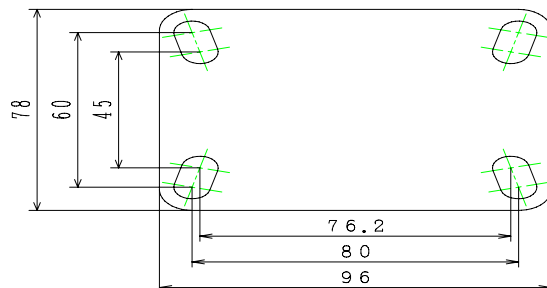
平板尺寸图:
